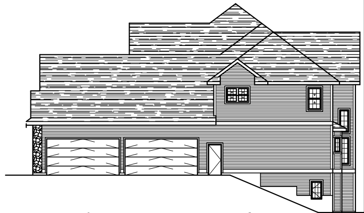
RIGHT ELEVATION
