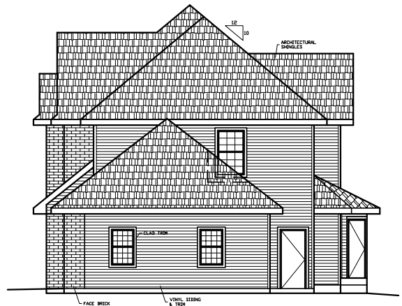
RIGHT ELEVATION
