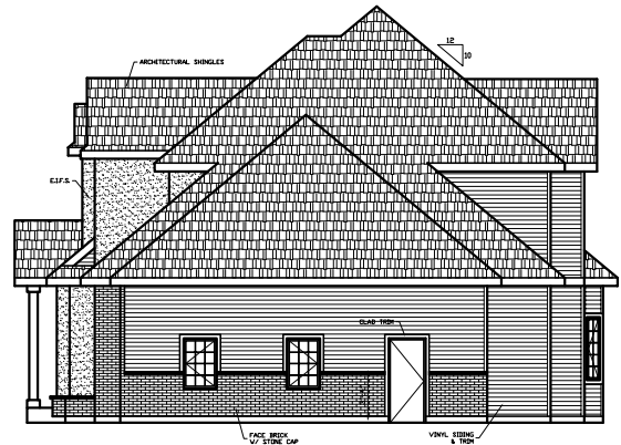
RIGHT ELEVATION
