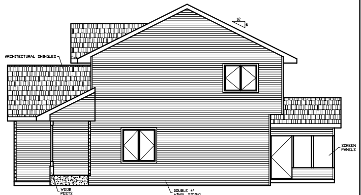
RIGHT ELEVATION
