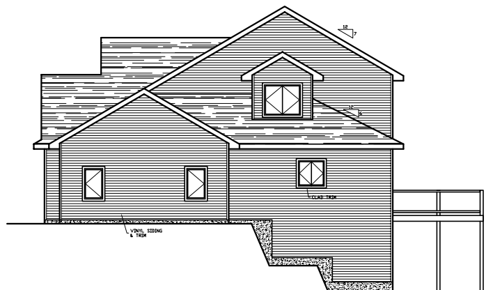
RIGHT ELEVATION
