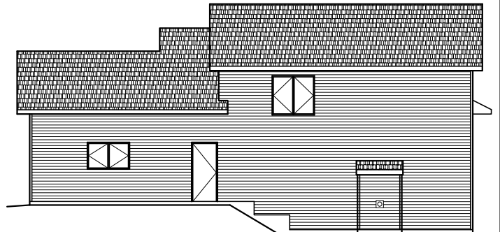
RIGHT ELEVATION
