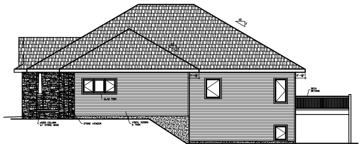
RIGHT ELEVATION
