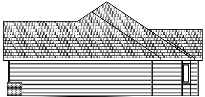
RIGHT ELEVATION
