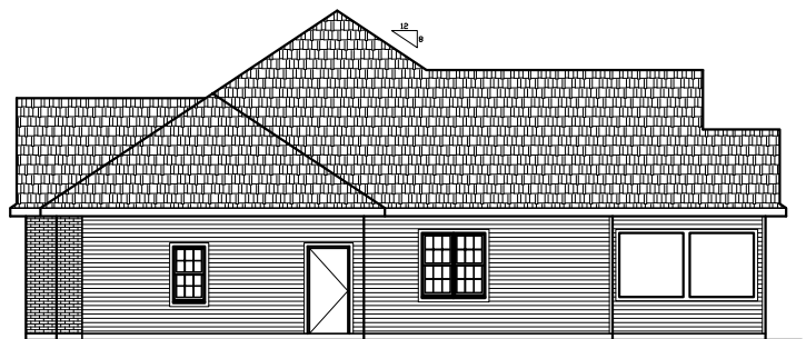
RIGHT ELEVATION
