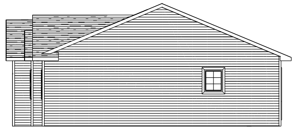
RIGHT ELEVATION
