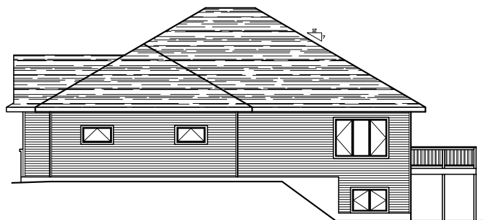
RIGHT ELEVATION
