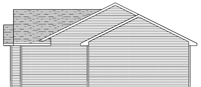
RIGHT ELEVATION
